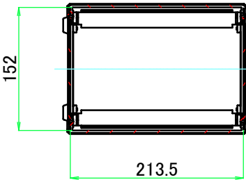
A-A ( 1 : 6.5 )
