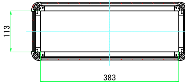
C-C ( 1 : 6.5 )
